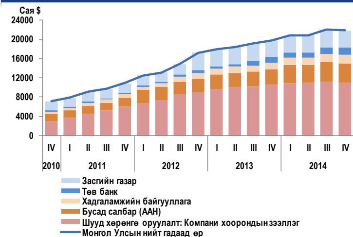
Дүрслэл 4. Статистик хамаарал
