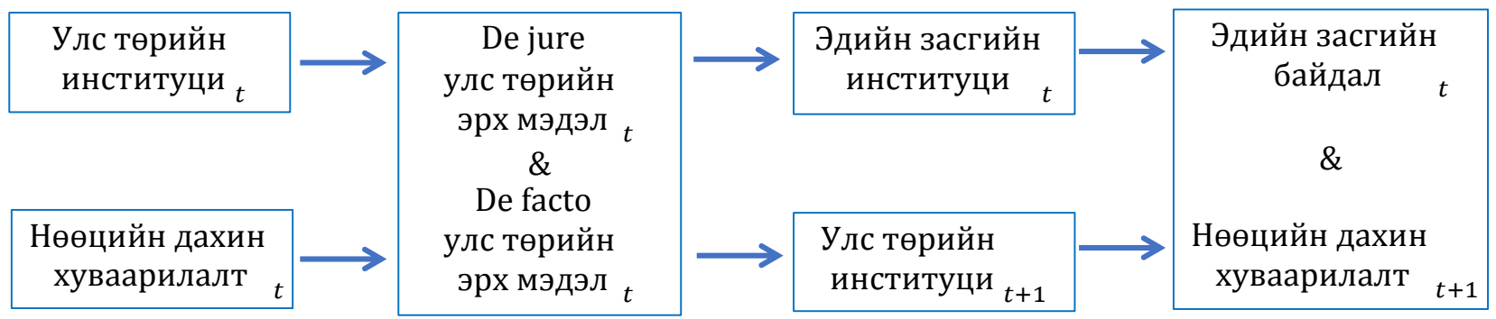
Эх сурвалж: Acemoglu and Robinson (2008)
